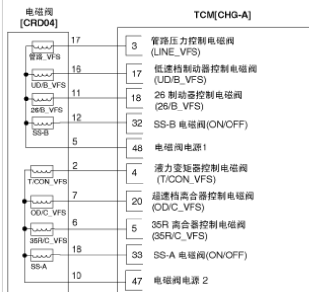
[电路图]
